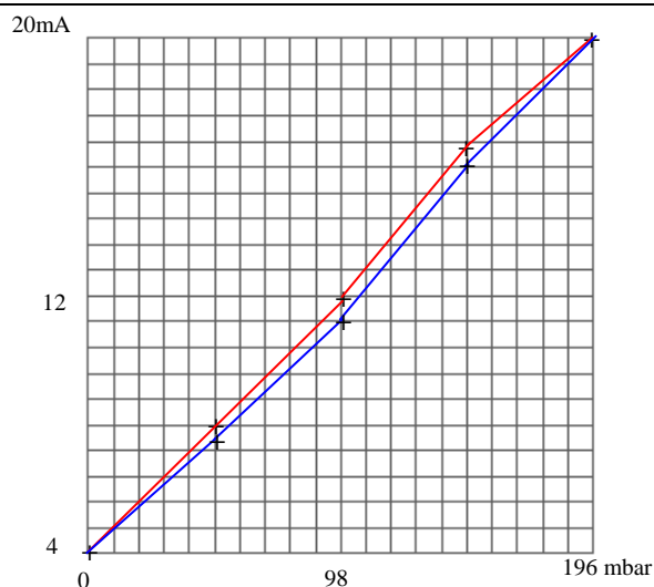
Korreksjon/kalibreringskurve
